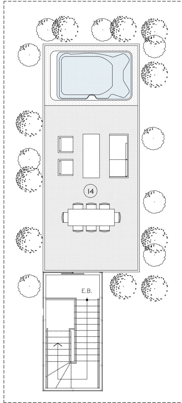
TOITURE
