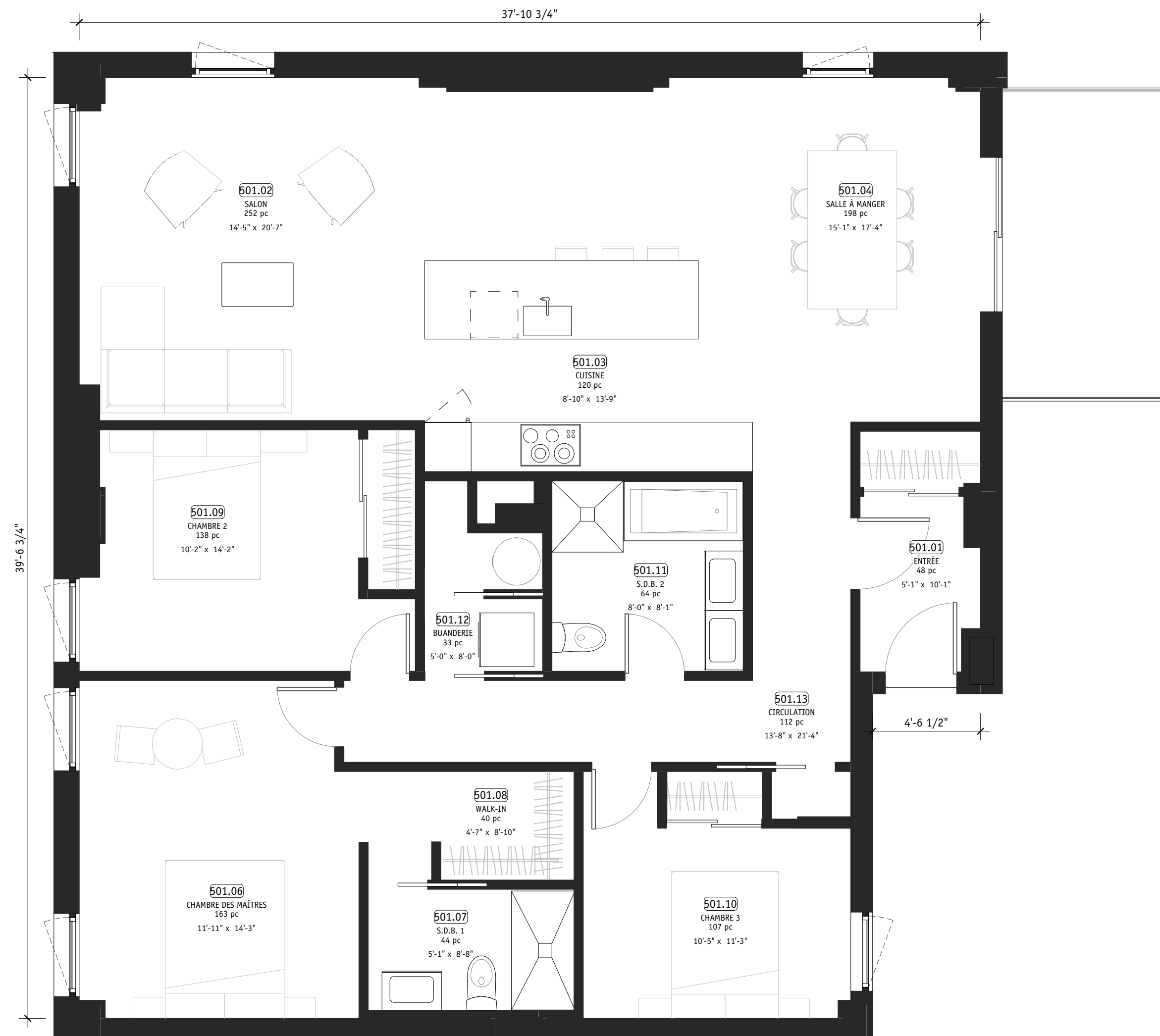
1 PLAN 501 - 5E ÉTAGE A161 1/4" = 1'-0"
